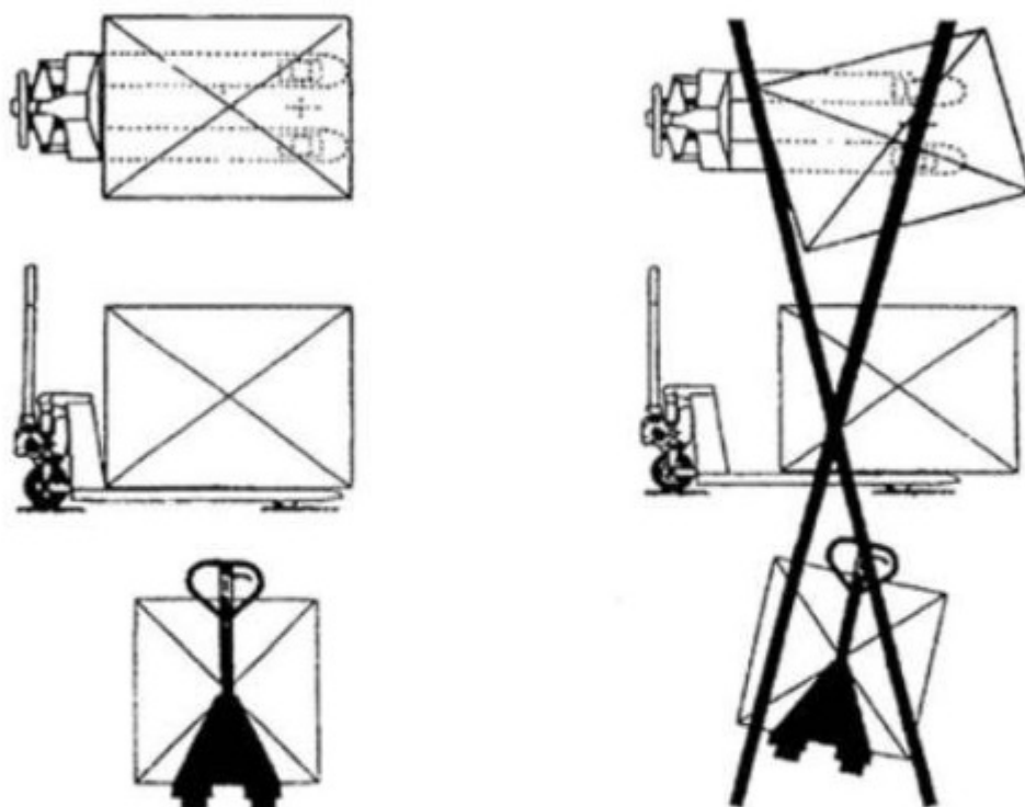
Рисунок 7. Схема расположения груза на вилах
