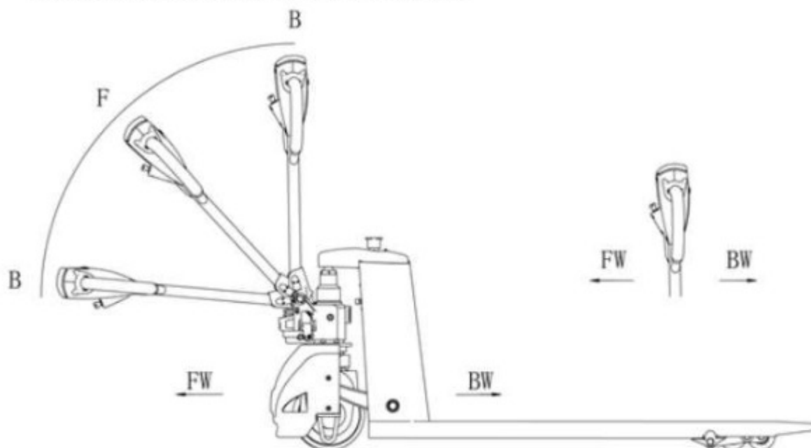
Рисунок 5. Управление тележкой.
